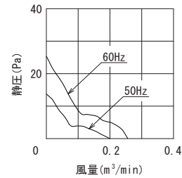
風量～静圧特性曲線
